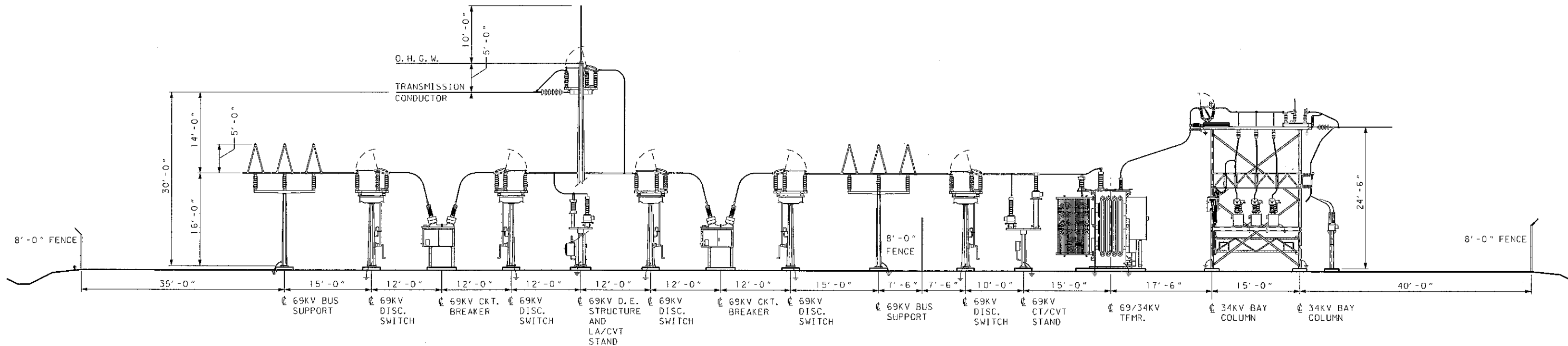
ELEVATION A-A
